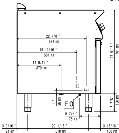
Oldalnézet
